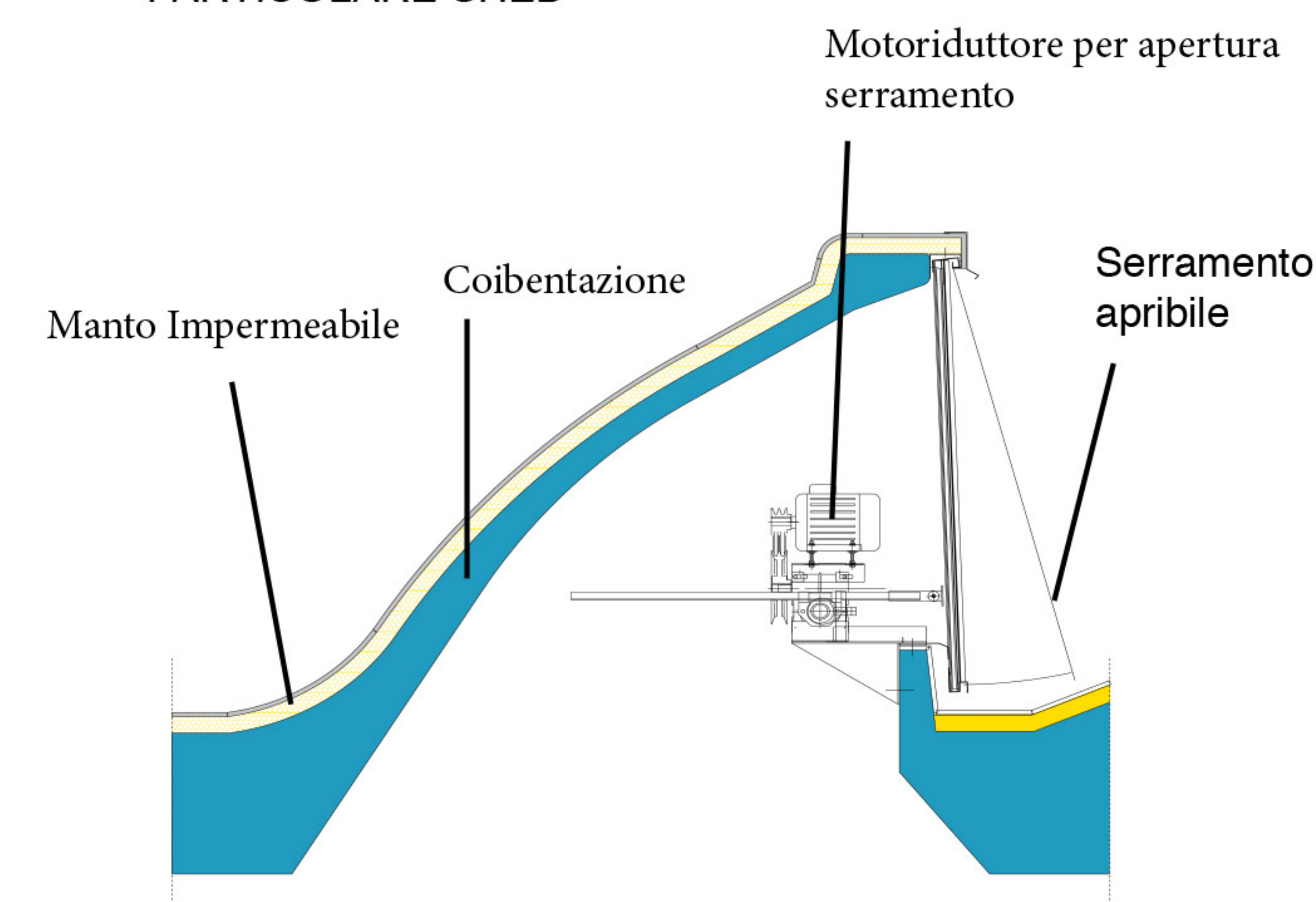
PARTICOLARE SHED
