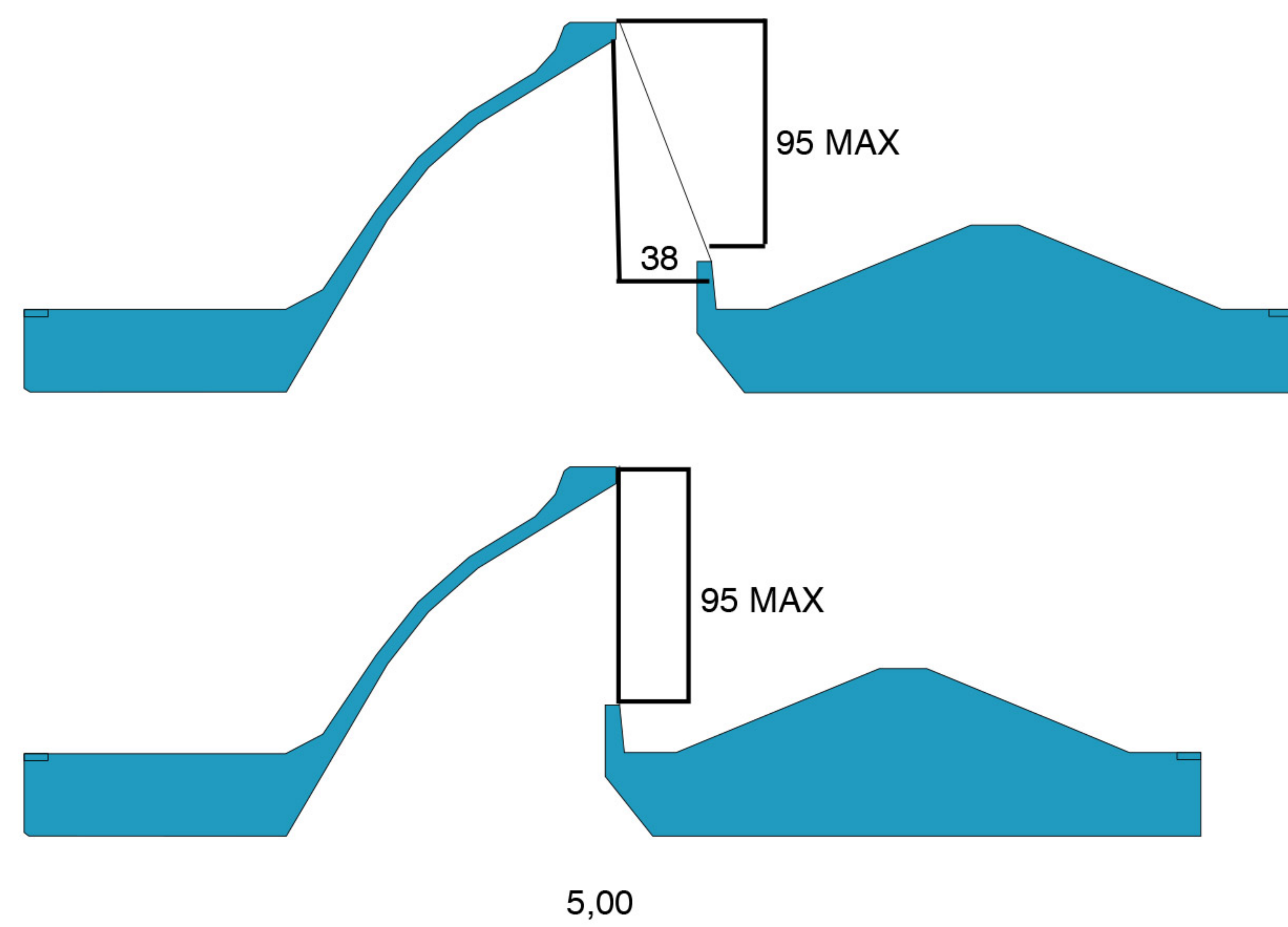
LA COMBINAZIONE "EUROCOP E SHED"
