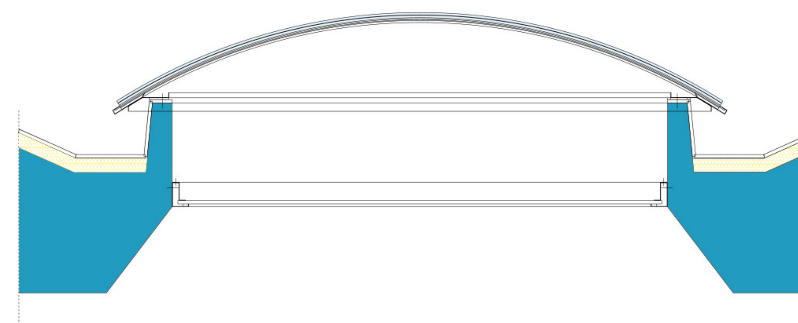
PARTICOLARE LUCERNARIO
